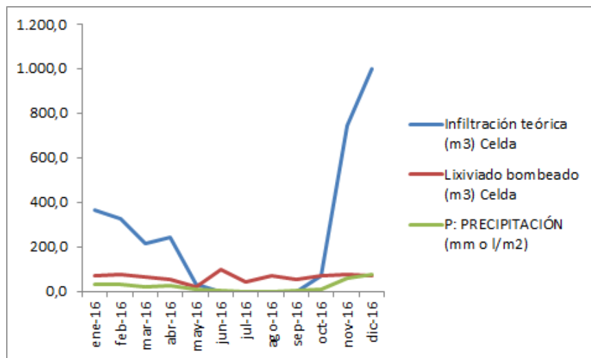
Hidrograma 2016
